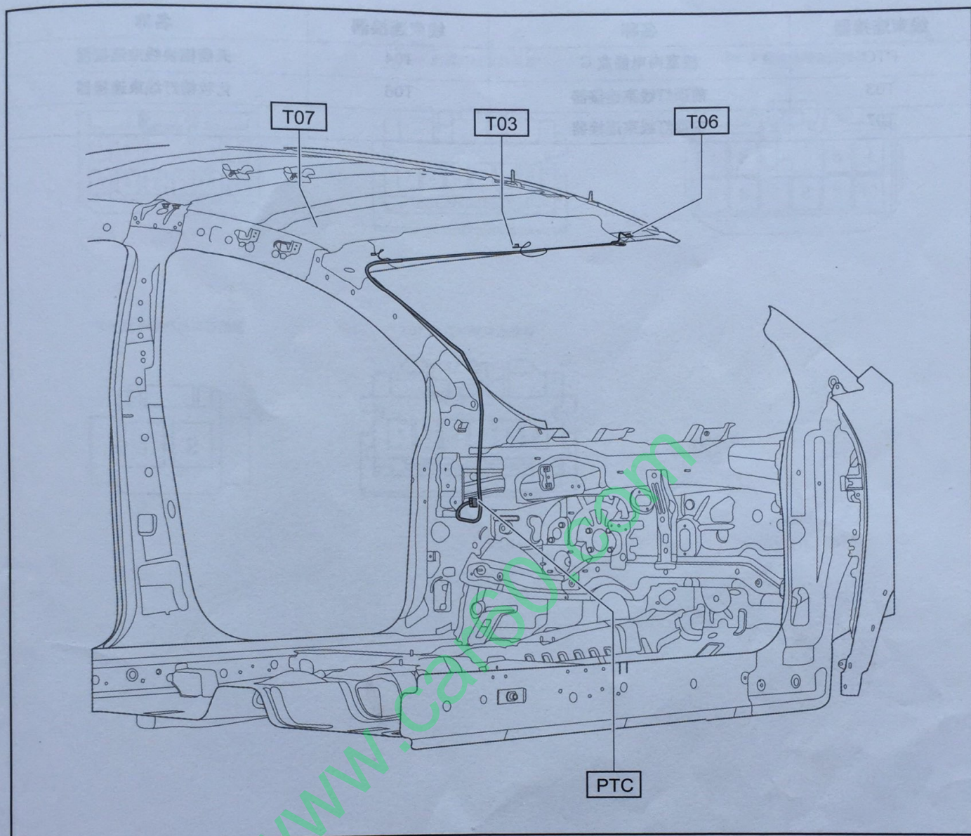
顶棚线束布置图
